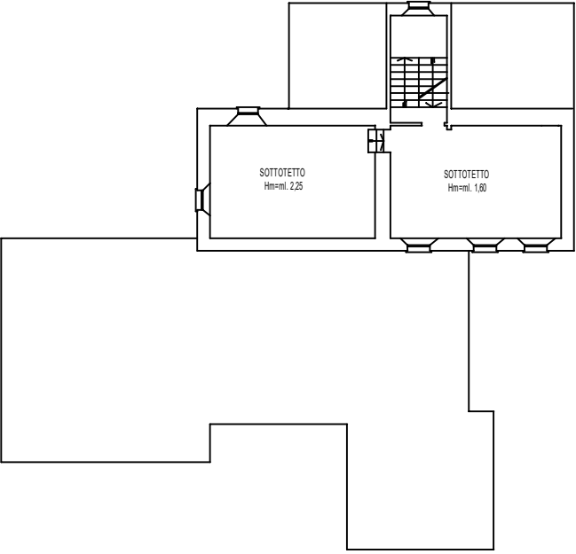
SECONDO PIANO
